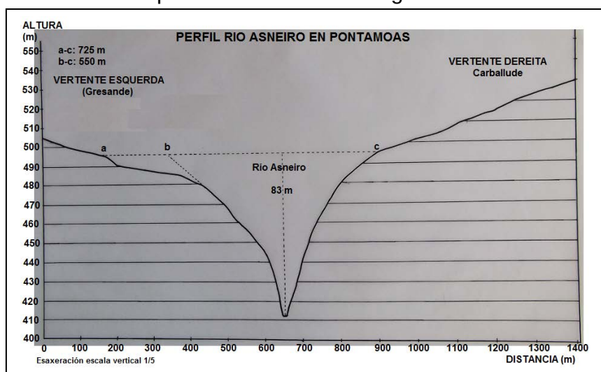
FIGURA 1.1 Perfil topográfico dunha sección do río Asneiro entre Pontamoas e a aldea de Carballude (Donsión). O lateral esquerdo corresponde á vertente esquerda (parroquia de Gresande) e o dereito a outra vertente (parroquia de Donsión).
