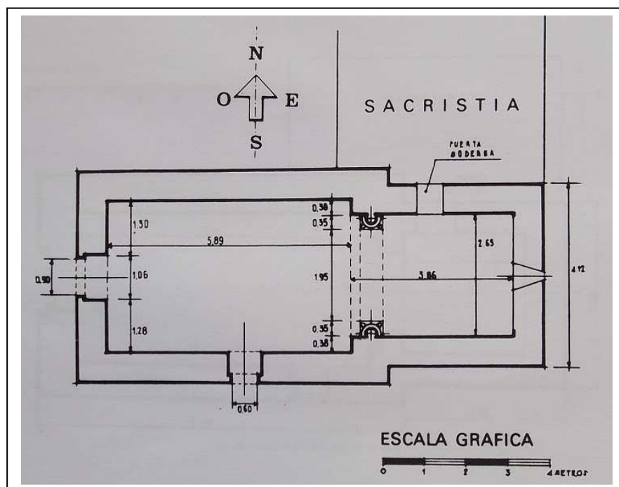
4.2 Plano de igrexa de Santa Baia. Bango Torviso
